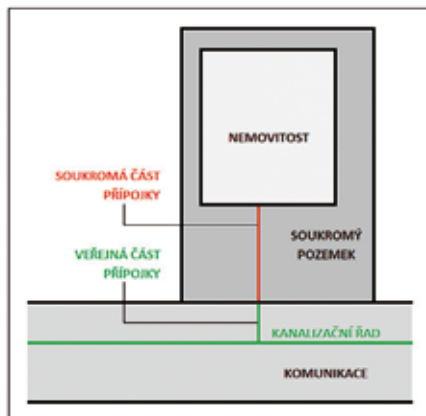
Schéma připojení nemovitosti na kanalizaci
