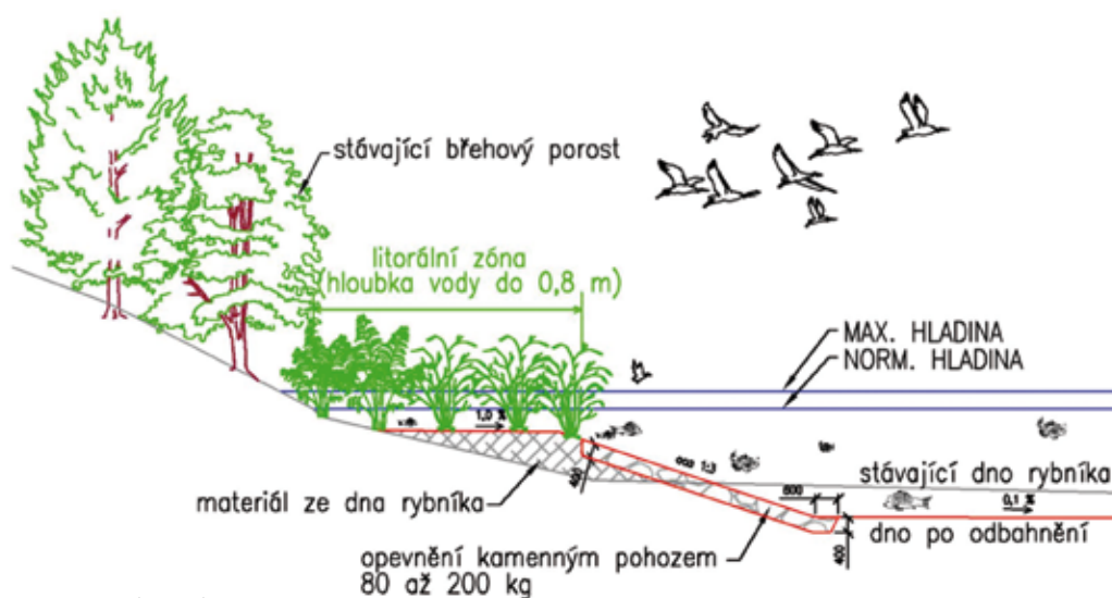
Vzorový řez litorální zónou
